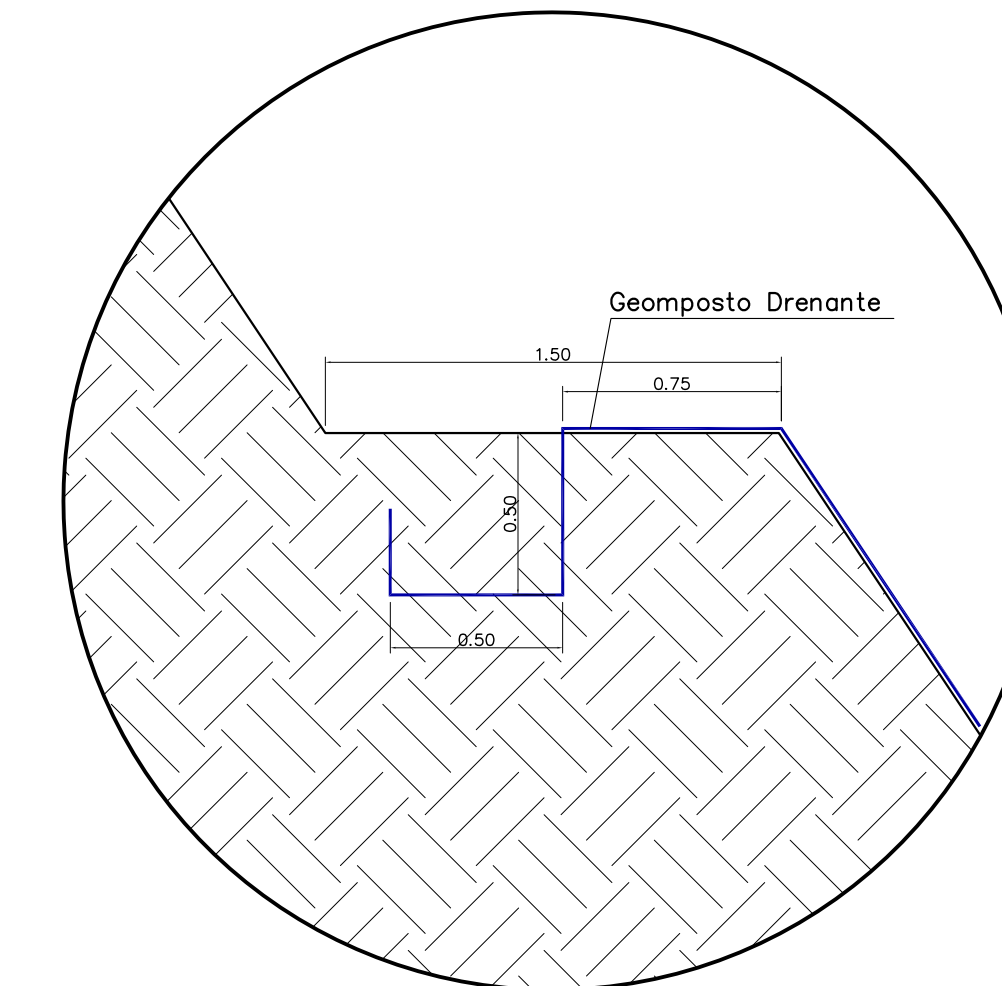
DETALHE DA ANCORAGEM DO GEOCOMPOSTO DRENANTE ESCALA 1:25
