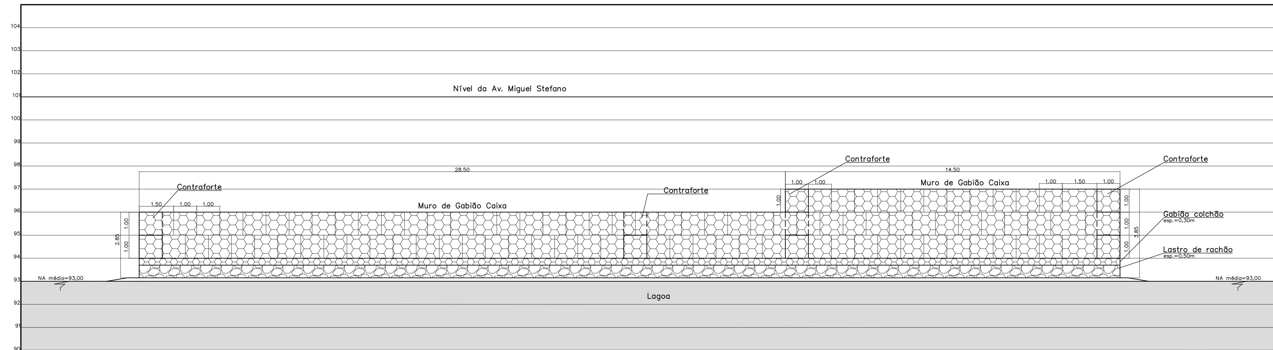
ELEVAÇÃO FRONTAL DO MURO DE GABIÃO ESCALA 1:100
